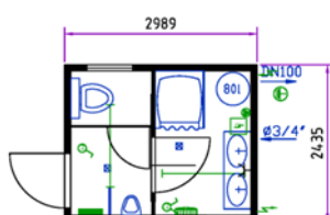
Bungalow sanitaire 10'
