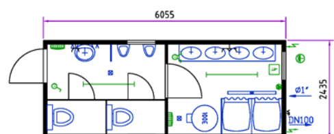
Bungalow sanitaire 20'
