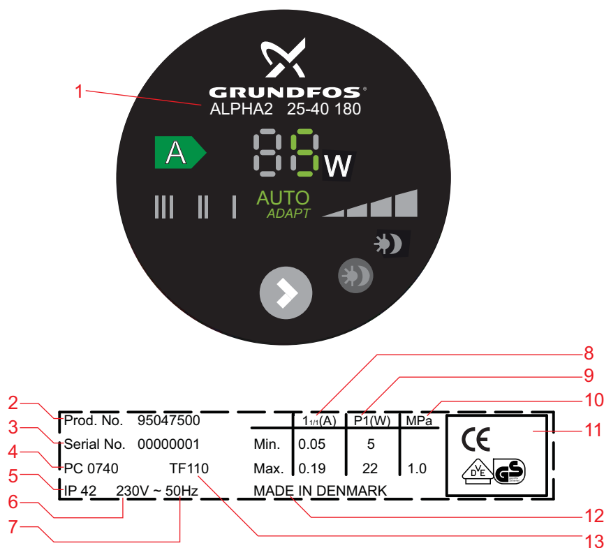
Fig. 21 Plaque signalétique, GRUNDFOS ALPHA2
