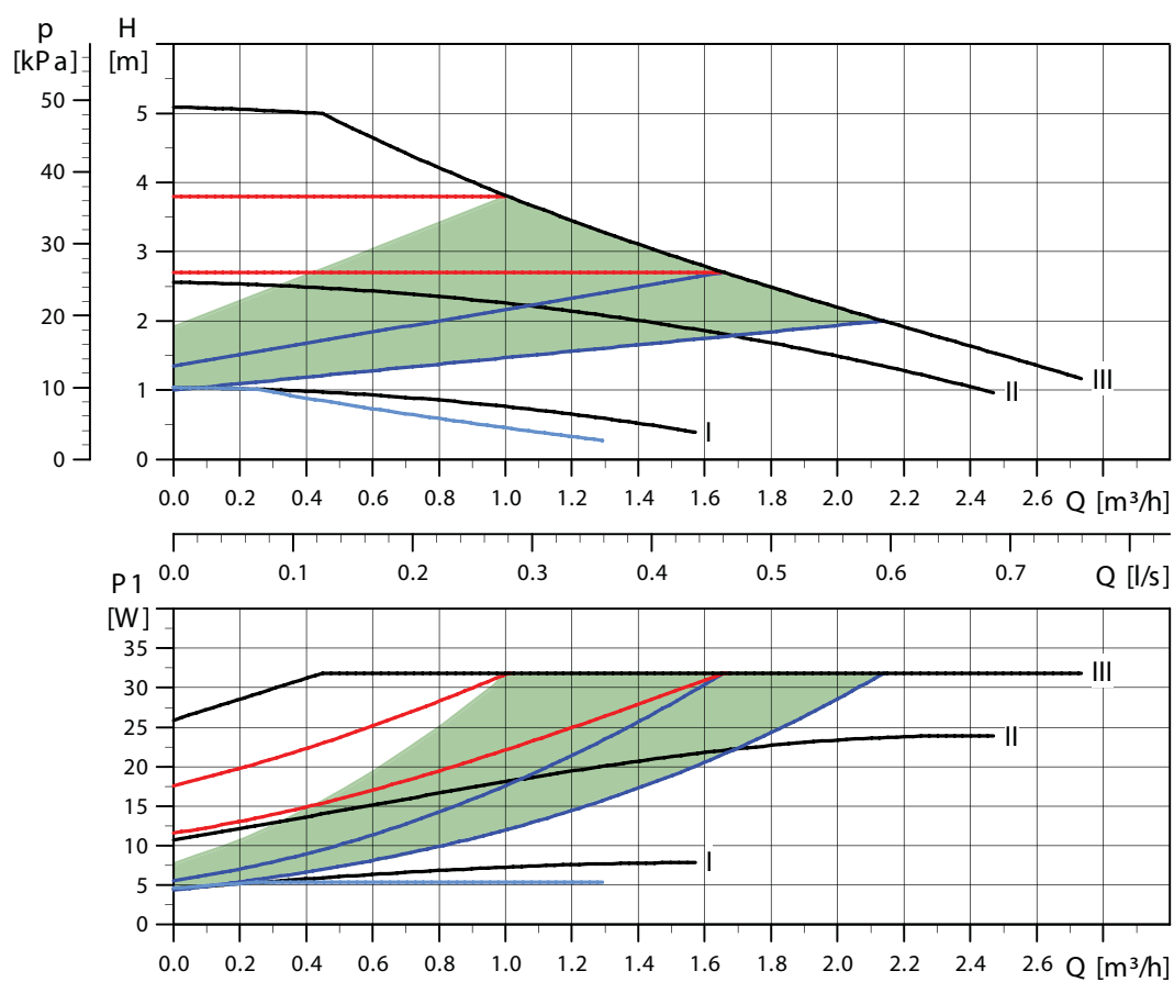
Fig. 19 Courbes de performances, ALPHA2 XX-50
