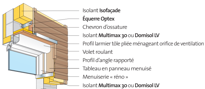
Solution 2 : Traitement du linteau pour panneau menuisé à base de bois, stratifié tôle ou lames de lambris avec menuiserie et volet roulant « réno »
