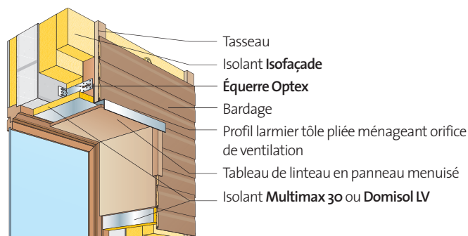
Solution 1 : Traitement du linteau par panneau menuisé à base de bois ou stratifié ou tôle avec menuiserie existante
