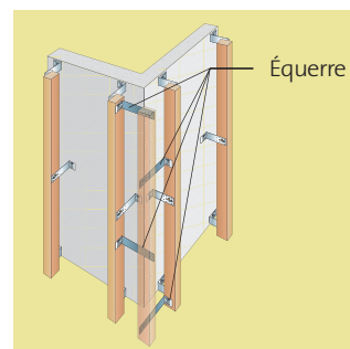
Solution 3 : Traitement ITE en deux couches avec fixation du chevron d'angle par équerre et plaque d'angle
